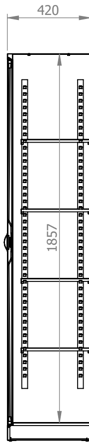
SECTION A-A 1 : 19
