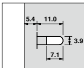
Seitbefestigung (mm)
