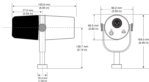
Gesamtabmessungen
