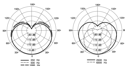
Typische Richtcharakteristik
