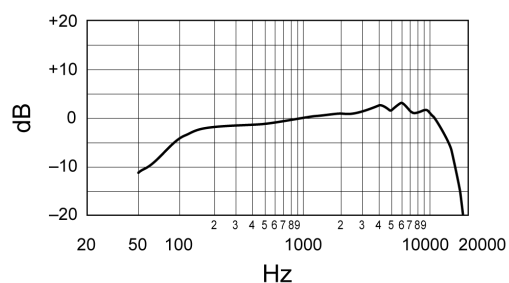
Typischer Frequenzgang
