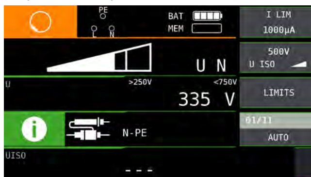
Anzeige Isolationsmessung
