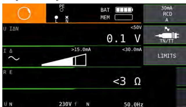
Anzeige RCD-Messung
