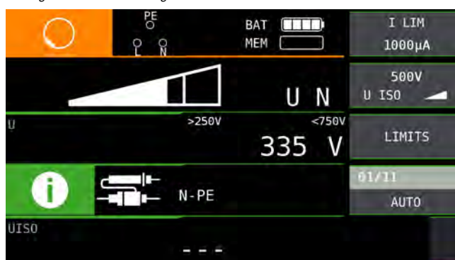
Anzeige Isolationsmessung
