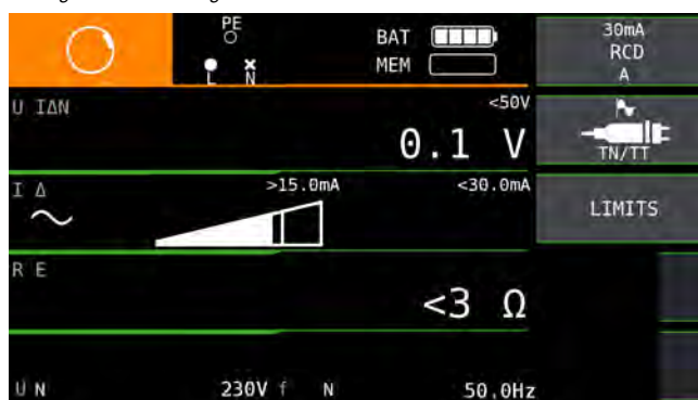
Anzeige RCD-Messung
