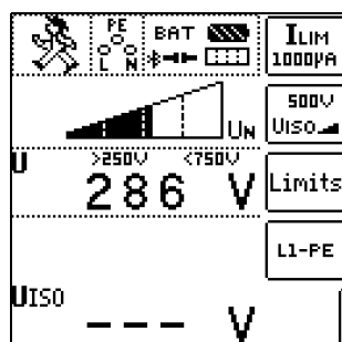
Isolationssmessung
