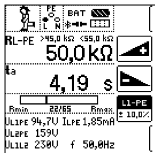
IMD-Prüfung
