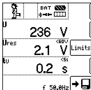
Restspannungsmessung
