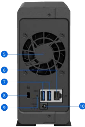
DS124 (Rückseite)
