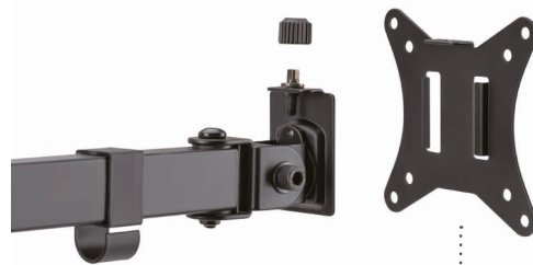
Detachable VESA plate
