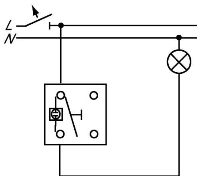
Aus 1-polig
