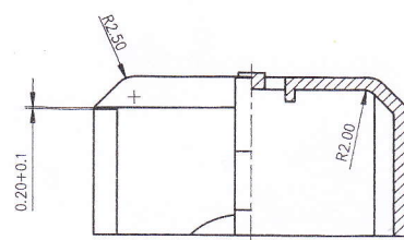
Schnitt C-D
