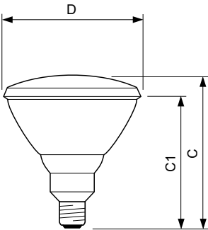
PAR38 IR 175W E27 230V Red
