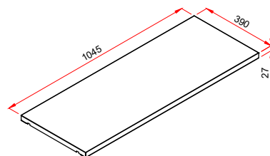
Fachboden
