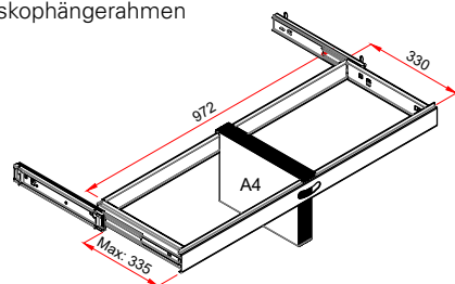
Teleskophängerahmen
