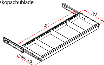
Teleskopschublade
