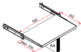
Teleskopboden
