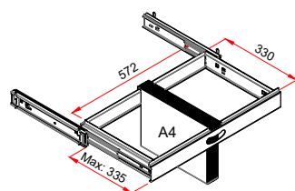
Teleskophängerahmen
