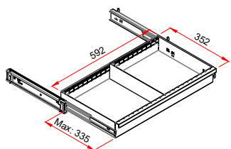
Teleskopschublade
