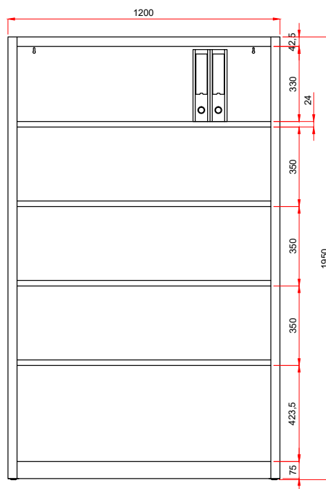
Frontansicht ohne Türen
