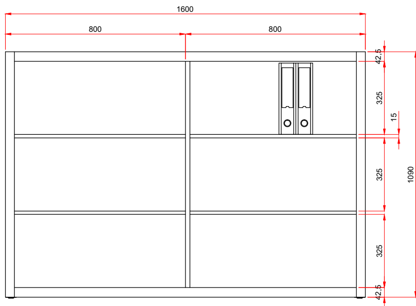
Frontalansicht - ohne Türen
