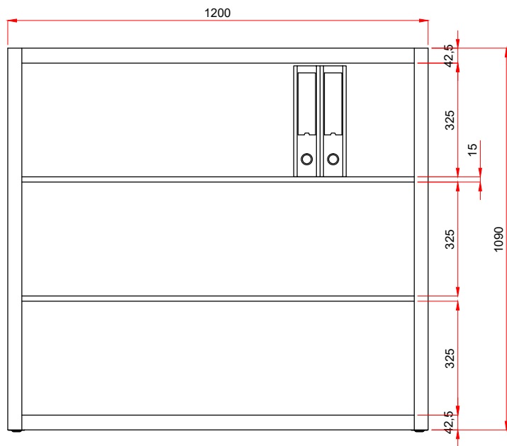
Frontalansicht - ohne Türen
