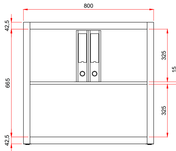
Frontalansicht ohne Türen
