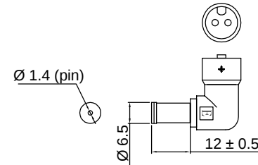
Adapterstecker 5 / Adapter plug 5 Typ „L“ / Type „L“ Material: PVC 20p, schwarz / Material: PVC 20p, black
