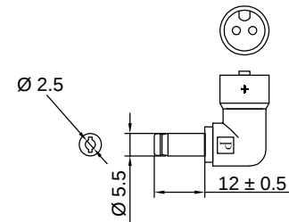
Adapterstecker 8 / Adapter plug 8 Typ „L“ / Type „L“ Material: PVC 20p, schwarz / Material: PVC 20p, black
