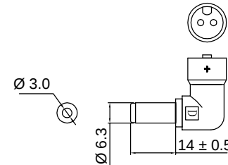
Adapterstecker 6 / Adapter plug 6 Typ „L“ / Type „L“ Material: PVC 20p, schwarz / Material: PVC 20p, black
