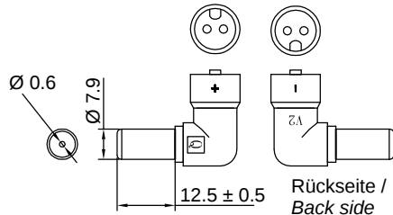
Adapterstecker 2 / Adapter plug 2 Typ „L“ / Type „L“ Material: PVC 30p, schwarz / Material: PVC 30p, black
