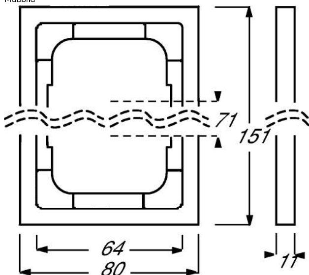
Maßbild
