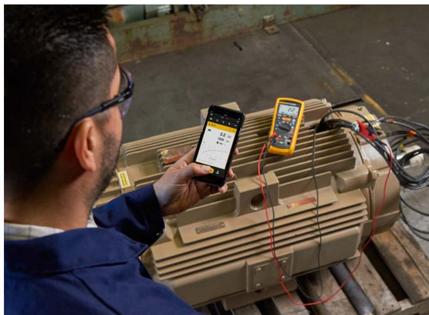
Datenspeicherung und gemeinsame Datennutzung über die Fluke-Connect-App beim Fluke 1587 FC
