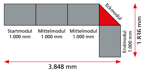
Außenmaße Theken-Set 2*
