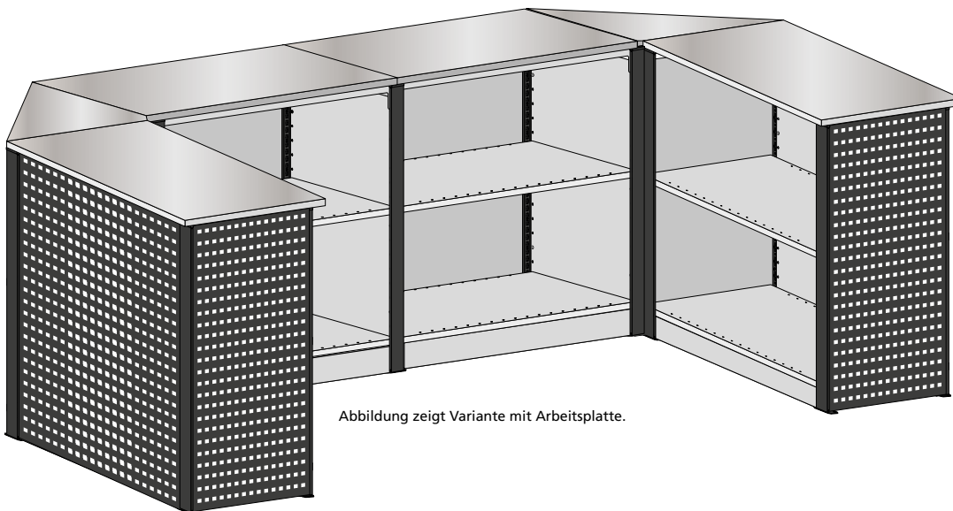
Außenmaße Theken-Set 3*
