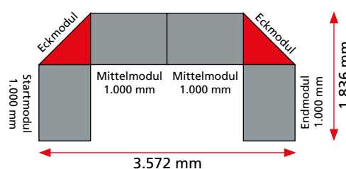
Außenmaße Theken-Set 3*
