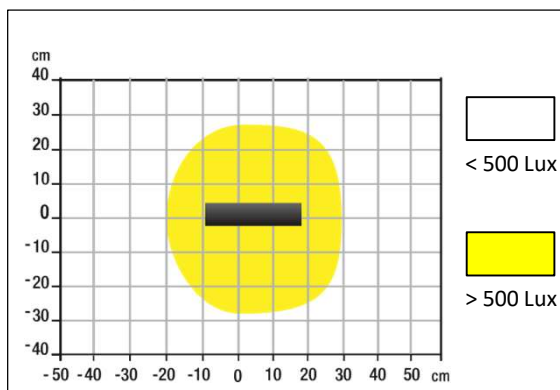
Lichtverteilungskurve, Draufsicht bei 35 cm Abstand:
