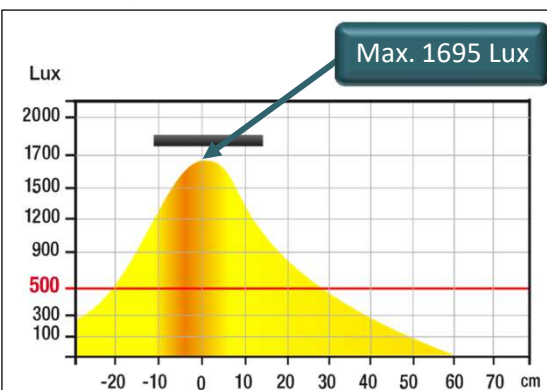
Lichtverteilungskurve, Seitenansicht bei 35 cm Abstand:
