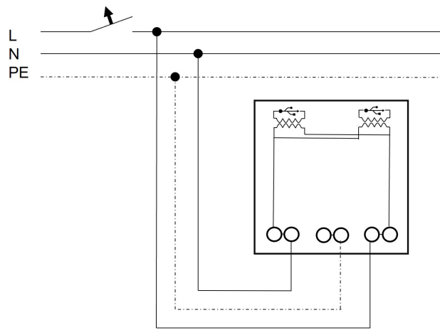
Anschlussbild
