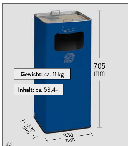
Abb.: Ascher/Abfallsammler B 32 R, enzianblau, Art.-Nr. 3083
