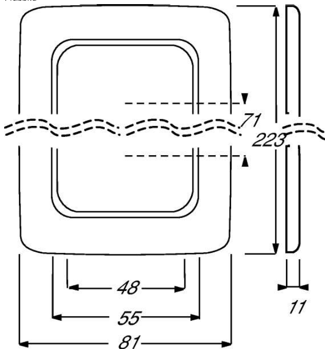
Maßbild
