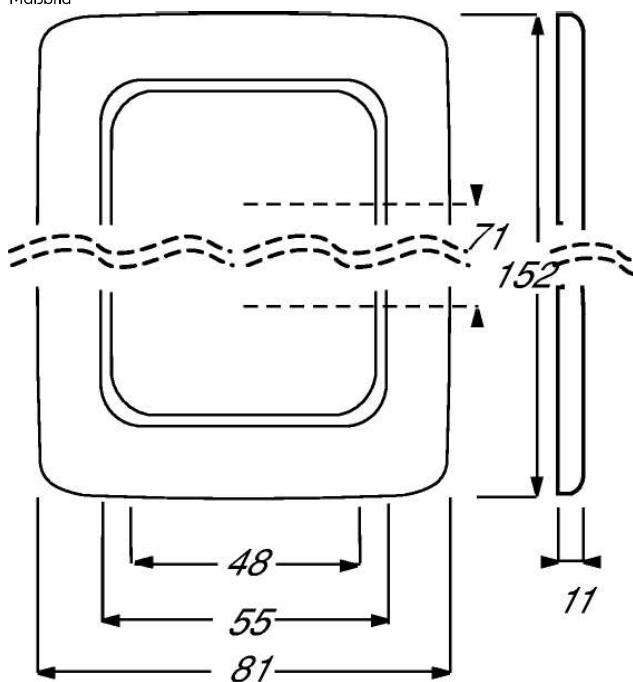
Maßbild
