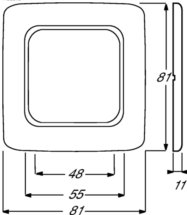
Maßbild
