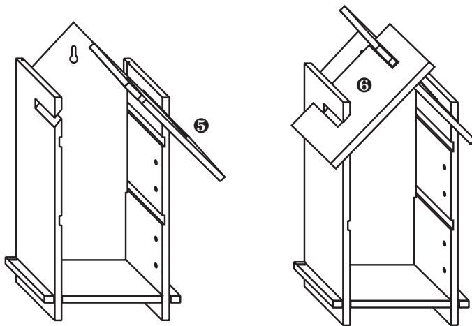
Montage Dach
