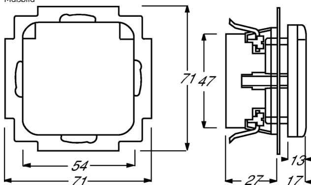
Maßbild
