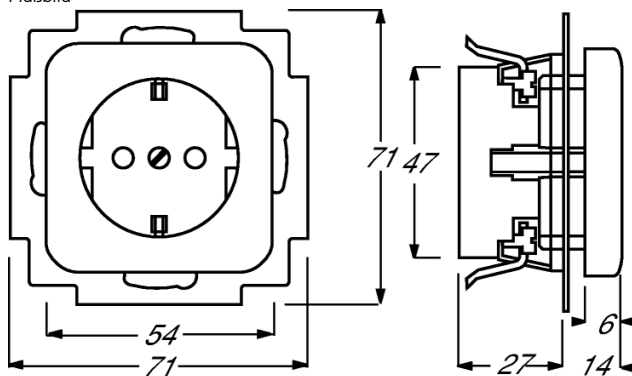
SCHUKO® Steckdose 20 EUC-21x
