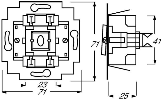
Maßbild
