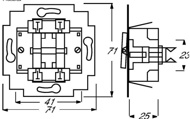
Maßbild
