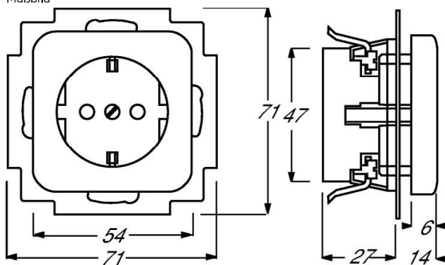
Maßbild
