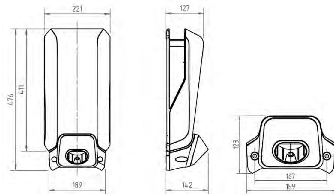
Abb. 1-1: Abmessungen in Millimeter
