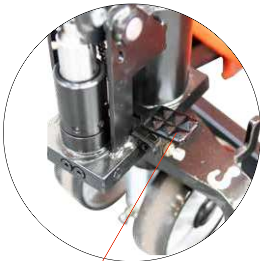
Fußablasshebel
