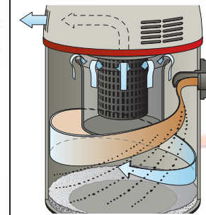
Die Grafik zeigt das patentierte Wasser-Abscheidesystem mit Zykloneinsatz Art.-Nr. 116.105
