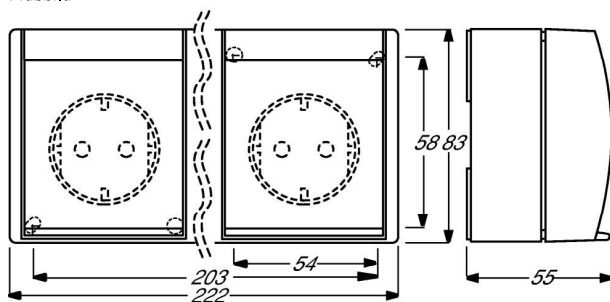
Maßbild
