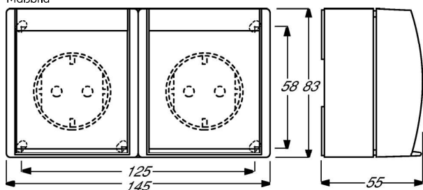
Maßbild
