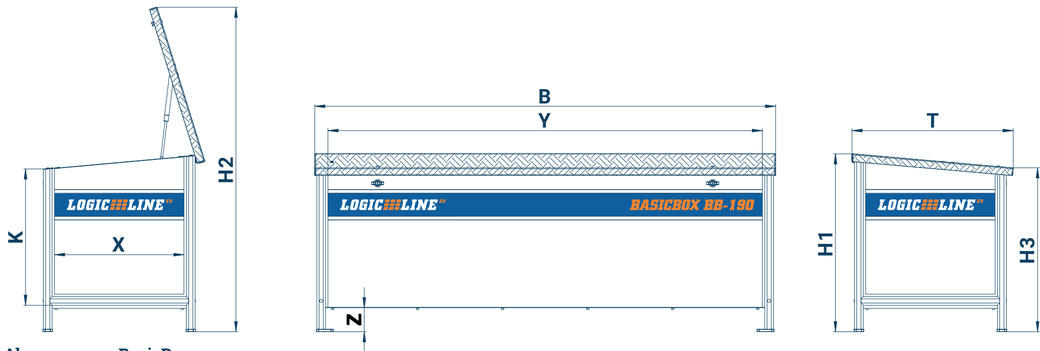
Abmessungen BasicBox
