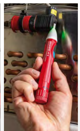
Prüfung eines Magnetventils
