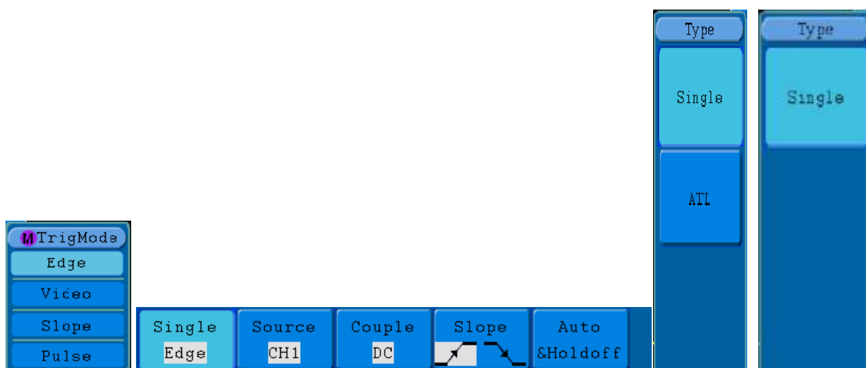
Fig. 29 Edge trigger menu
