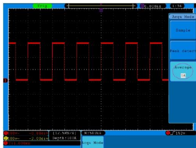
Abb. 40 die angezeigte Wellenform nachdem das Rauschen mit dem Average Mode entfernt wurde. Die Averagenummer wurde eingestellt auf 16.
