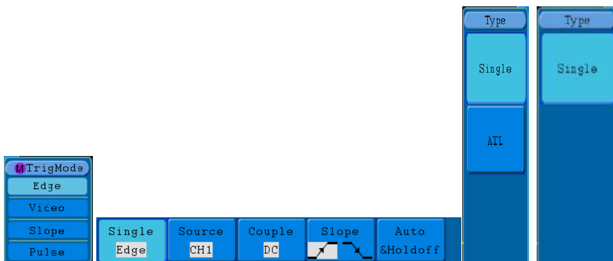
Fig. 30 Edge trigger menu
