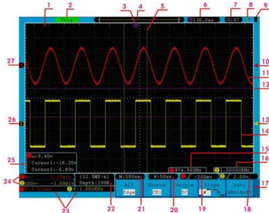
Abb. 6 Benutzeroberfläche
