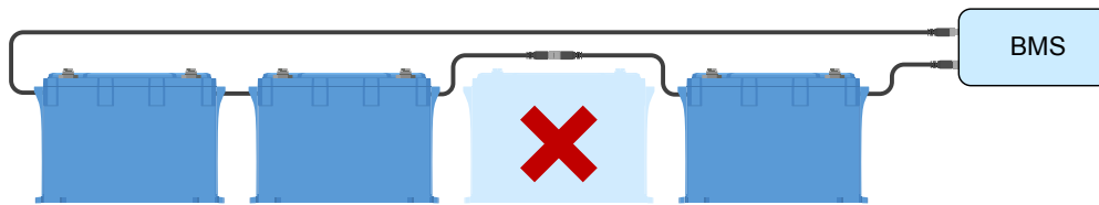
Eliminieren eines BMS-Fehlers durch Umgehen einer verdächtigen Batterie
