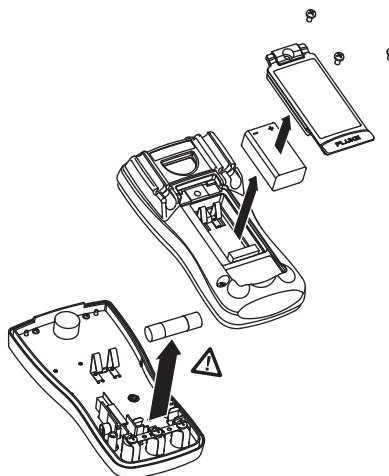
Abbildung 2. Demontage
