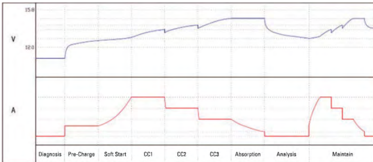
Abb.5-1: Ladezyklus Batterieladegerät
