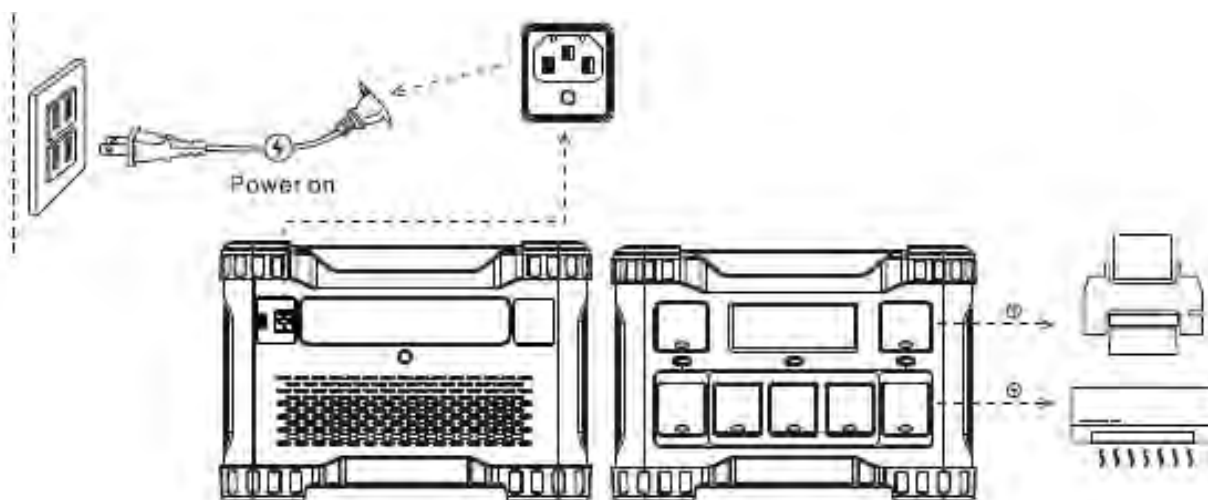
Abb.5-1: USV Funktion
