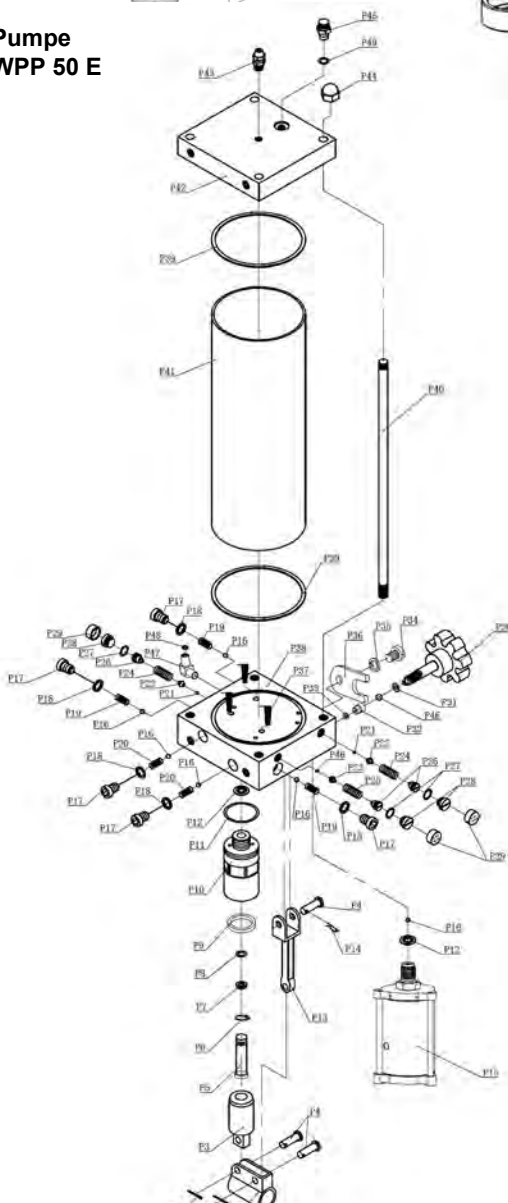
Abb. 26: Zylinder der hydraulischen Werkstattpresse WPP 20 E (oben links), WPP 30 E (oben Mitte), WPP 15 E (oben rechts); WPP 50 E und WPP 75 E (unten rechts); Pumpe WPP 50 E (unten links)
