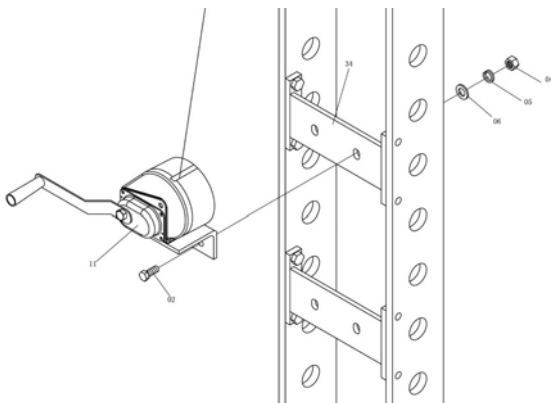
Abb. 10: Seilwinde montieren
