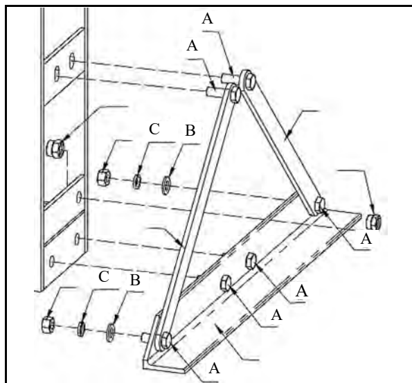
Abb. 8: Querfuß montieren
