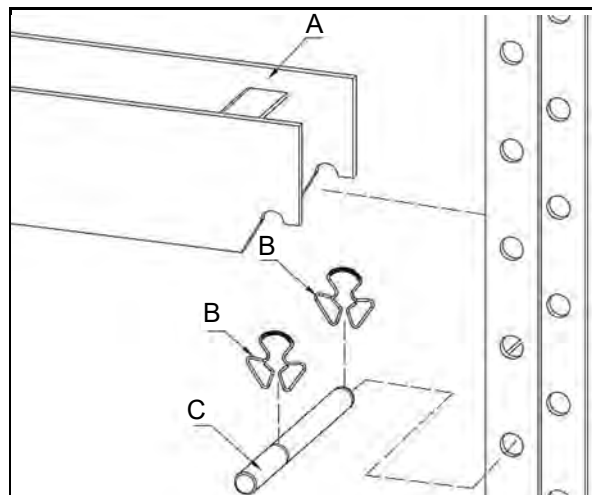
Abb. 9: Presstisch montieren
