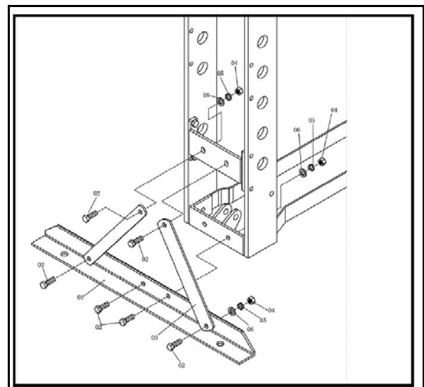
Abb. 9: Querfuß montieren
