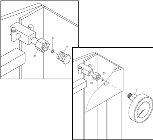
Abb. 7: Manometer montieren
