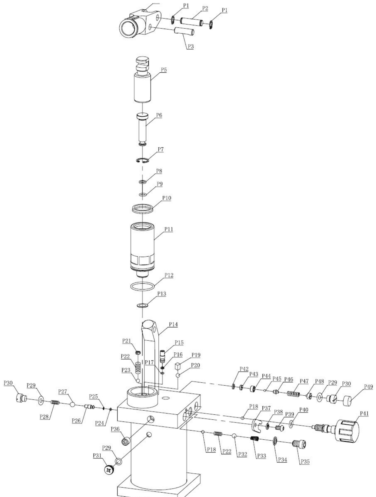
Abb. 11: Ersatzteilzeichnung 3
